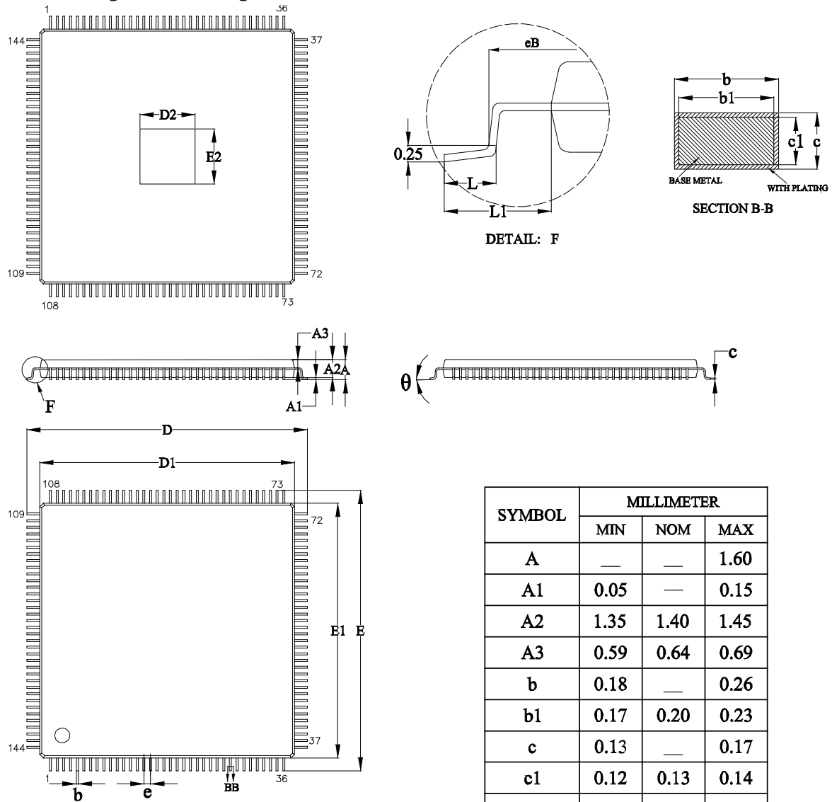
Figure 4-3 Package Outline EQ144/EQ144P/EQ144PF
