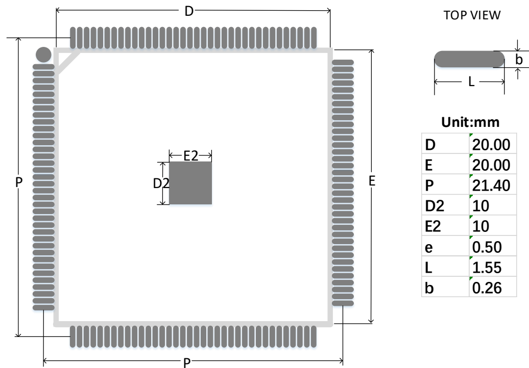
Figure 4-4 Recommended PCB Layout EQ144/EQ144P/EQ144PF
